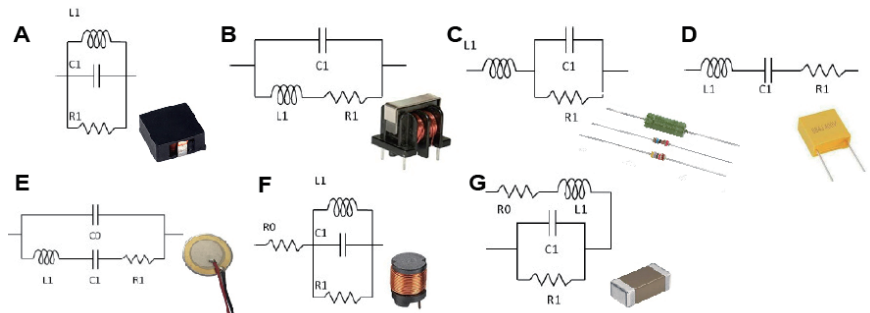
等效電路模型分析
