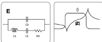
等效電路模型分析
